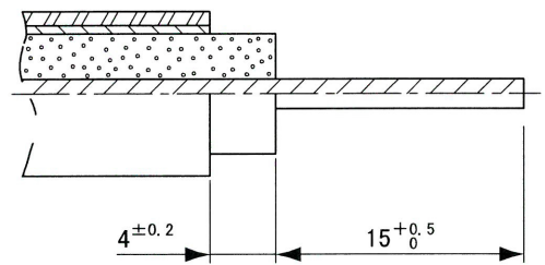
ケーブル切出し寸法
