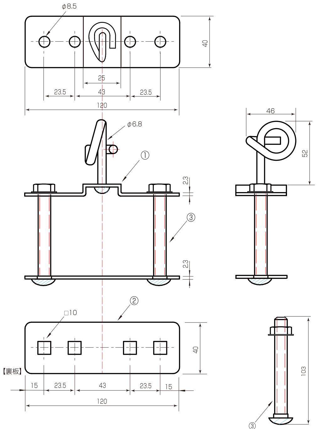
【根角ボルト】 附属品 M8×100mm/2本
