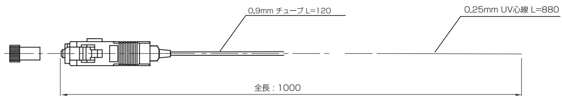
UV 心線の構造
