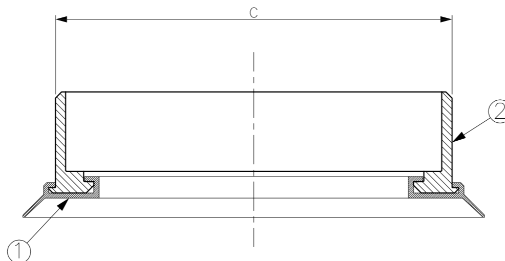
A-A' 断面
