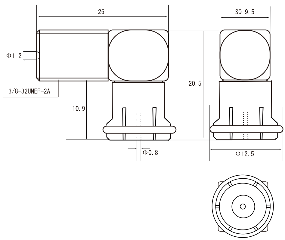
規格表 CFA-SL32 ストレートプラグ-メス端子
