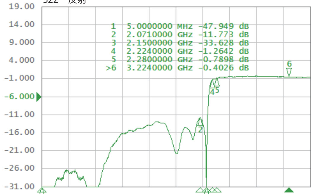
S22 反射
